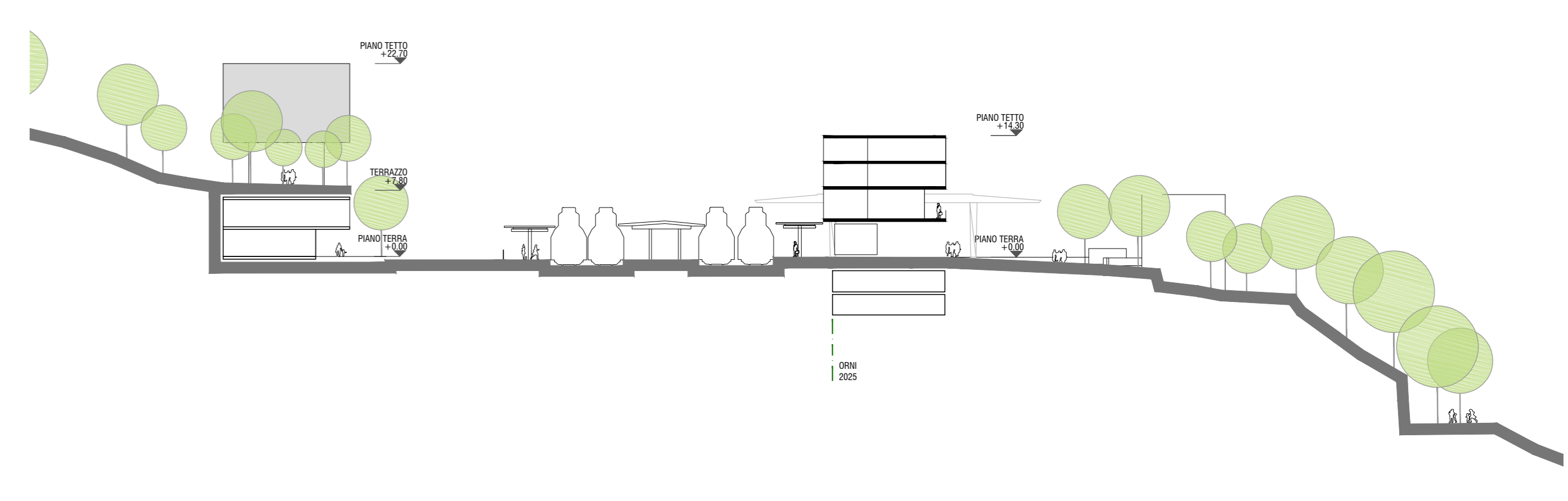
SEZIONE TRASVERSALE CC 1/500
