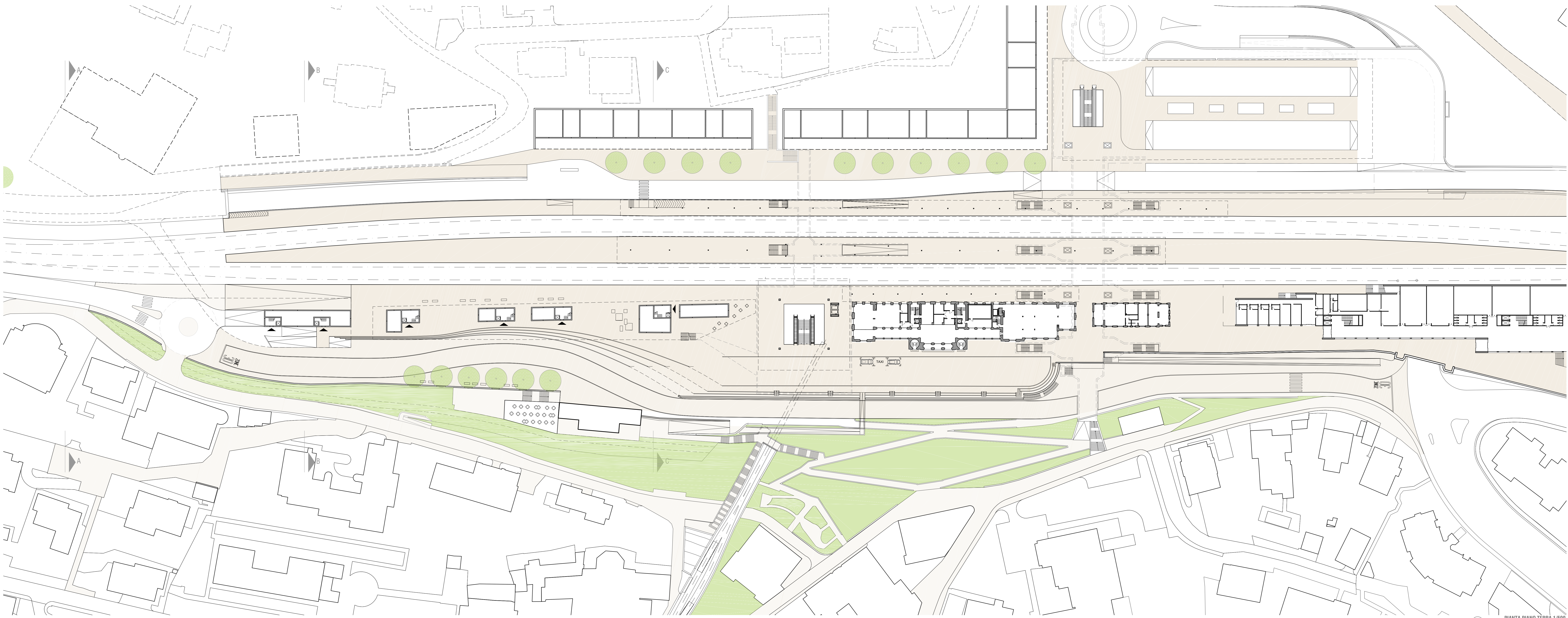
PIANTA PIANO TERRA 1/500
